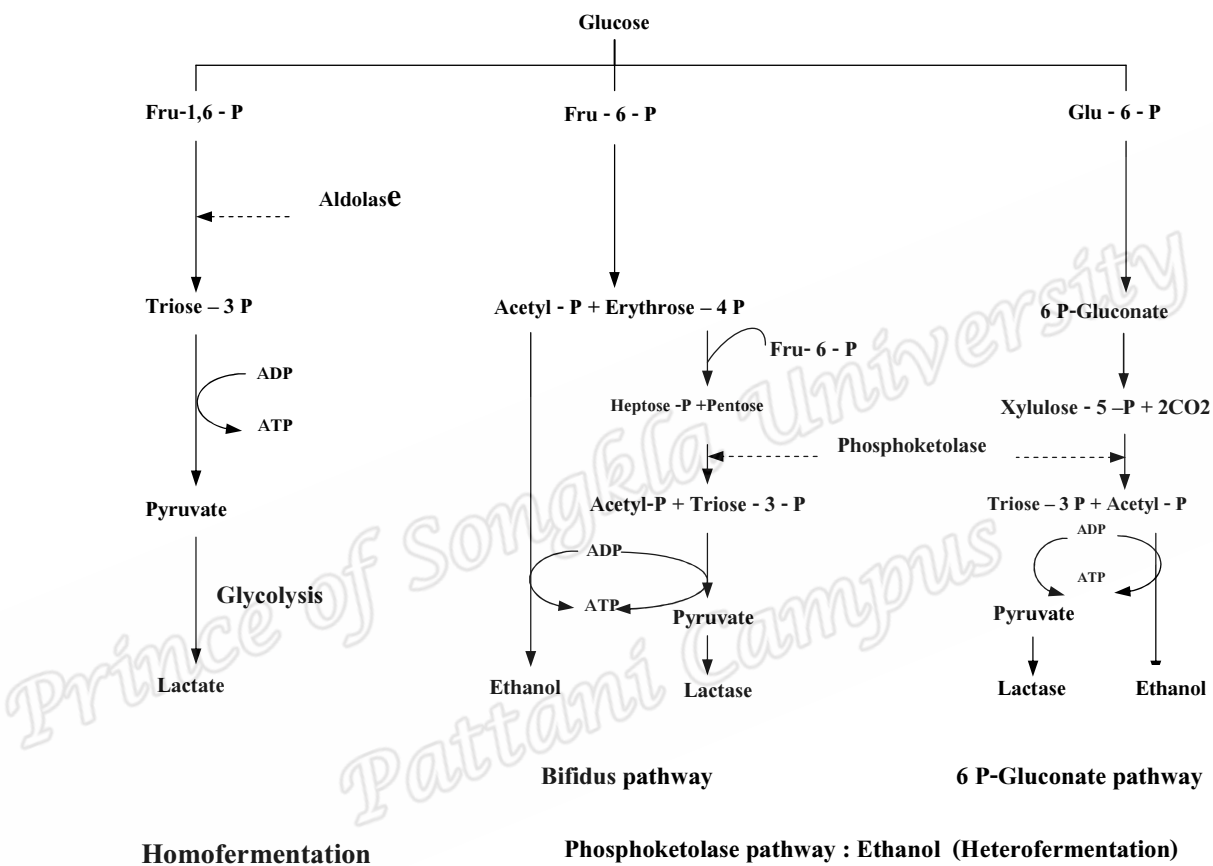
รูปที่ 1 รูปแบบการเปลี่ยนแปลงสารในกระบวนการหมักของแบคทีเรียกรดแลคติก ที่มา : Wood and Holzapfel (1995) อ้าง โดย กุณฉีกา (2547)
