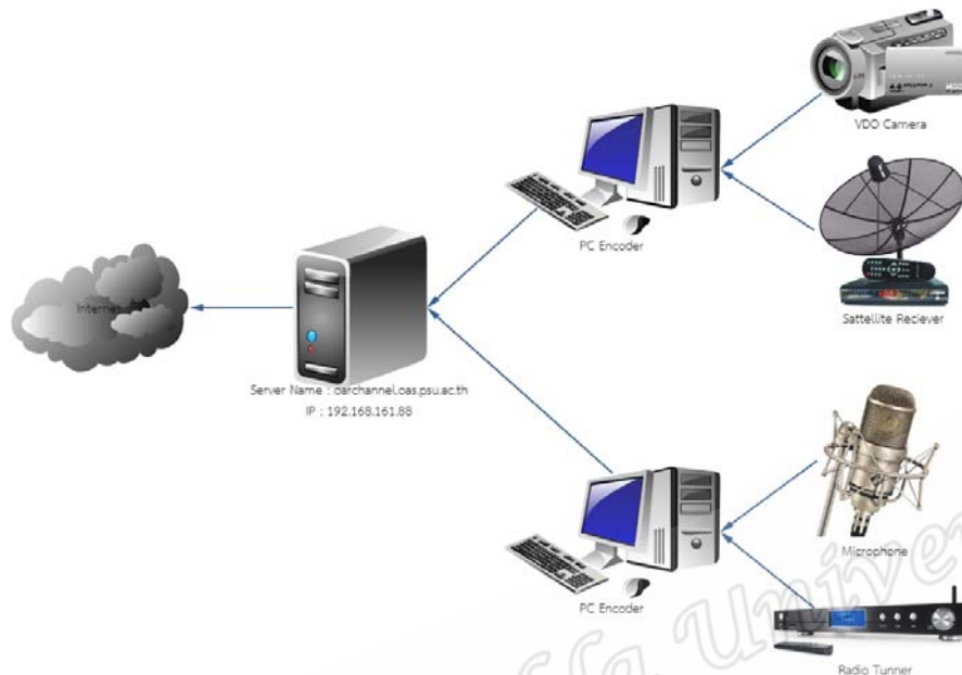
ภาพที่ 4.2 แผนผังแสดงกระบวนการรับส่งสัญญาณภาพและเสียงของสถานีวิทยุโทรทัศน์ผ่านเครือข่ายอินเทอร์เน็ตของสำนักวิทยบริการ มหาวิทยาลัยสงขลานครินทร์ วิทยาเขตปัตตานี
