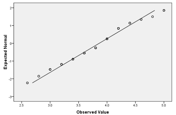
Normal Q-Q Plot of วัดและประเมิน
