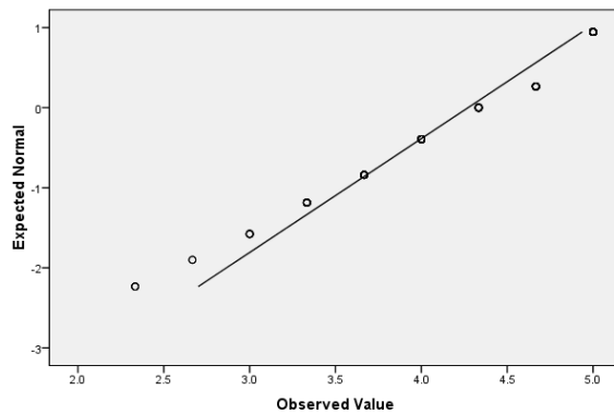
Normal Q-Q Plot of ปัจจัยด้านผู้ปกครอง
