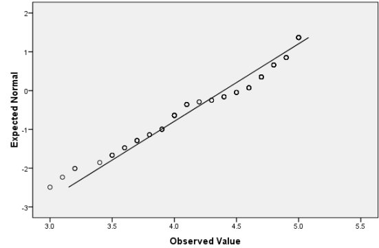
Normal Q-Q Plot of คุณลักษณะของครู
