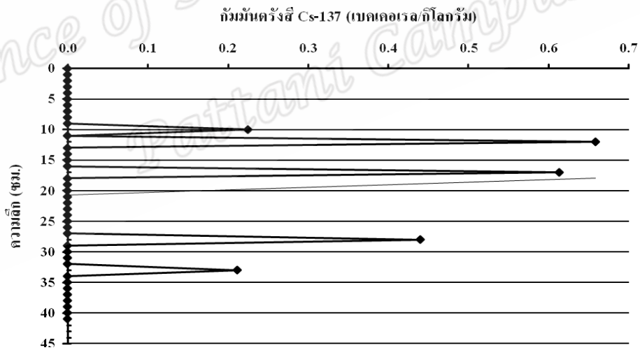
รูปที่ 4 แสดงความสัมพันธ์ระหว่างค่ากัมมันตรังสี Cs-137 กับระดับความลึกตะกอนดิน ณ สถานีบ้านดาไ้ะ
